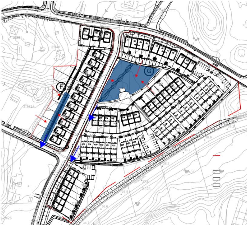
Figur 7. Instängda områden inom område FG är markerade med blått. Röda pilar redovisar avrinningen mot de instängda områdena. Blå pilar visar utlopp från de instängda områdena.
