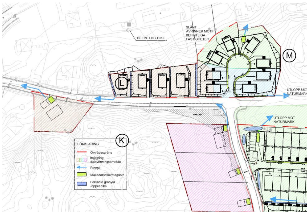
Figur 22 Föreslagen dagvattenhantering för kvarter K, L och M.
