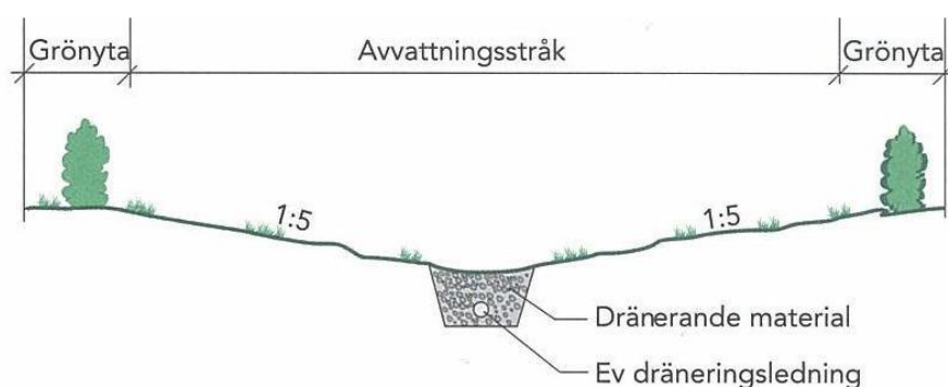
Figur 15 Avskärande stråk mellan tomtmark där avvattningsstråk krävs
