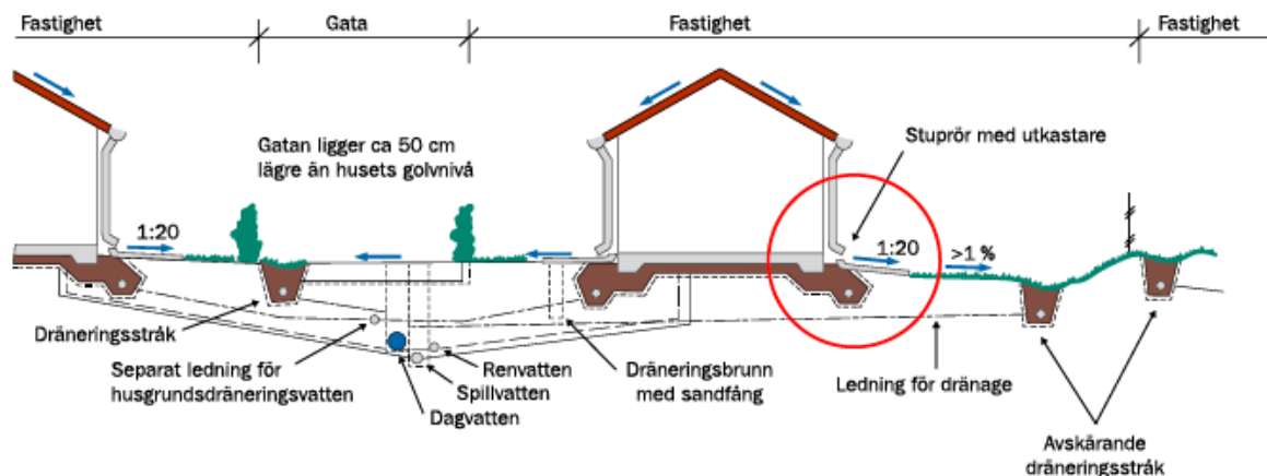
Figur 12. Föreslagen princip för att hantera kvartersmarkens dagvatten. Lokalgatorna kompletteras med dräneringsstråk längs med båda sidor av lokalgatan. Bild från Hållbar dagvattenhantering, Haninge kommun.
