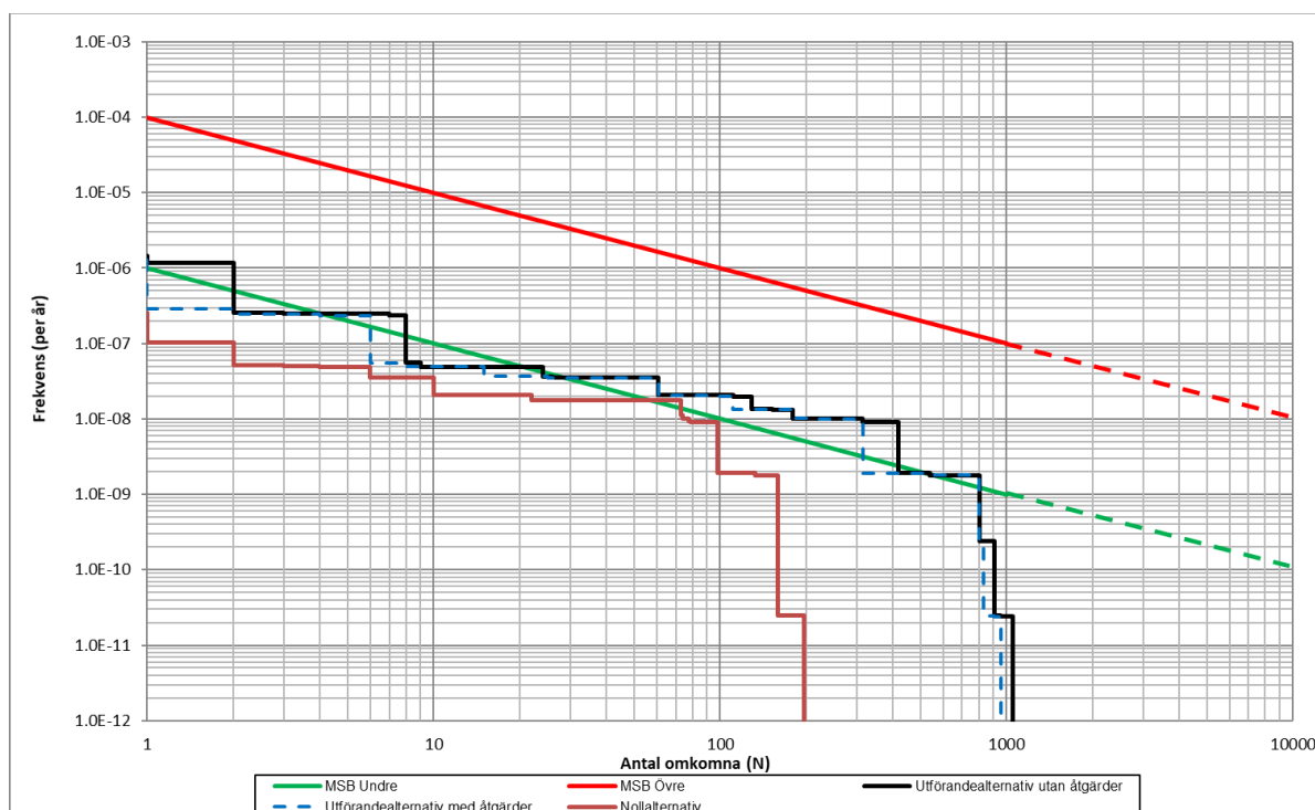
Figur C.4. F/N-kurva som redovisar samhällsrisknivå med avseende på skadescenarier på Nynäsbanan i Jordbro för studerat utförandealternativ utan , respektive, med rekommenderade restriktioner och åtgärder. Prognosår 2040.
