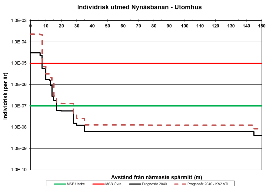
Figur C.6. Individrisk för oskyddad person utomhus som funktion av avståndet från Nynäsbanan (mätt från närmaste spårmit efter utbyggnad). Känslighetsanalys 2 – Förändrad beräkningsmetodik.
