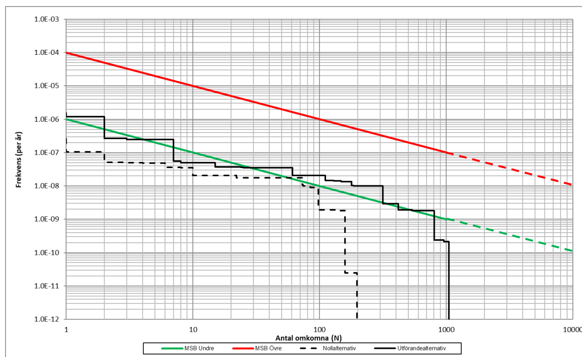
Figur C.3. F/N-kurva som redovisar samhällsrisknivå med avseende på skadescenarier på Nynäsbanan i Jordbro.
