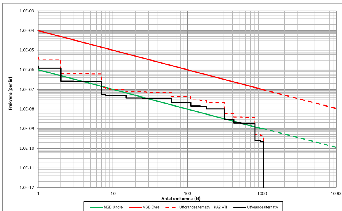
Figur C.7. F/N-kurva som redovisar samhällsrisknivån med avseende på skadescenarier på Nynäsbanan i Jordbro
