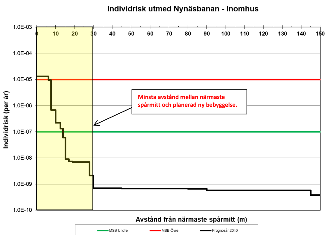
Figur C.2. Individriskprofil för person inomhus som funktion av avståndet från Nynäsbanan (mätt från närmaste spårmit).
