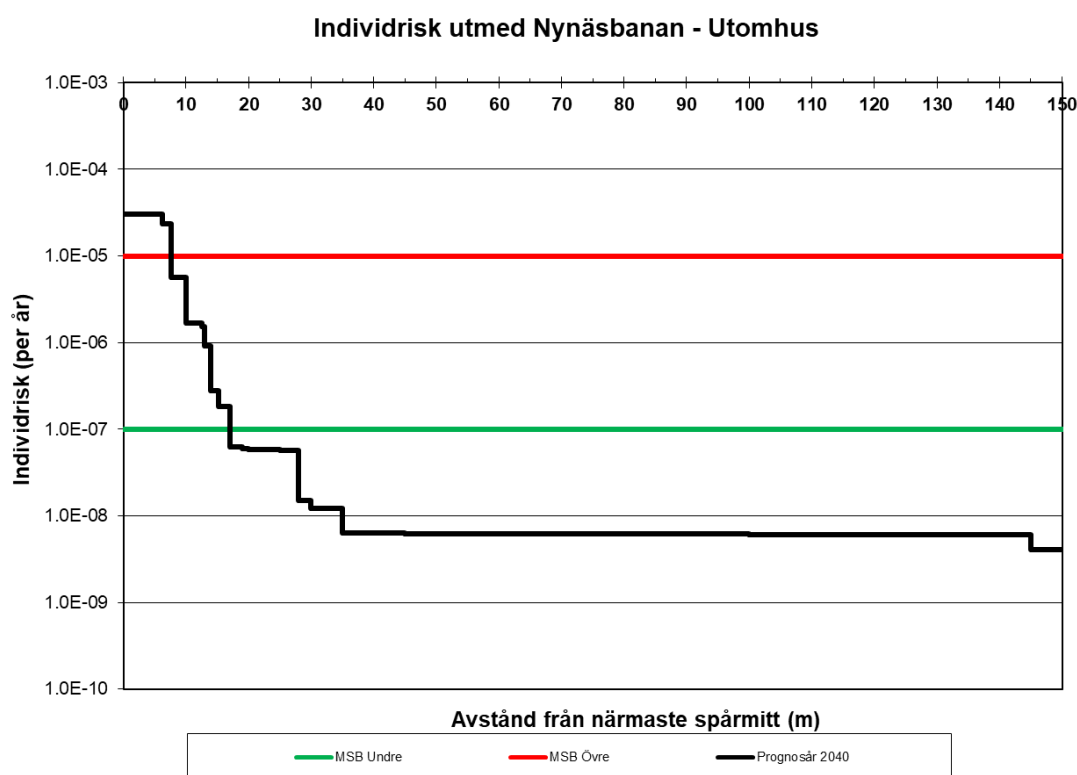
Figur C.1. Individriskprofil för person utomhus som funktion av avståndet till Nynäsbanan (mätt från närmaste spårmitt).
