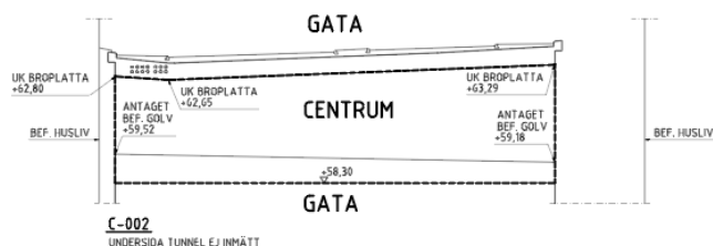
Bild 1.8-1.9. Planområdet och uppmätta höjder inom 3D-utrymmet i tvärsnitten A-002, B-002, C-002 och D-002. Sektionsritningarna visar utrymmet där centrumändamål (C) och markreservat för underjordiska ledningar (u) gäller.
