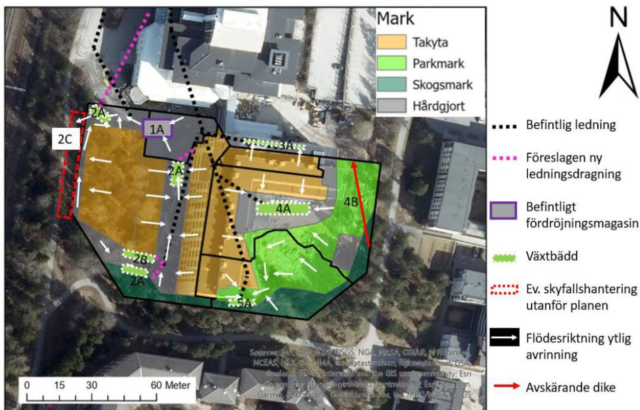
Figur 20. Föreslagen dagratten- och skyfallsshantering. Bild Afry. Observera att 2C ersätts av lösning med magasin beskriver under avrinningsområde 2.
