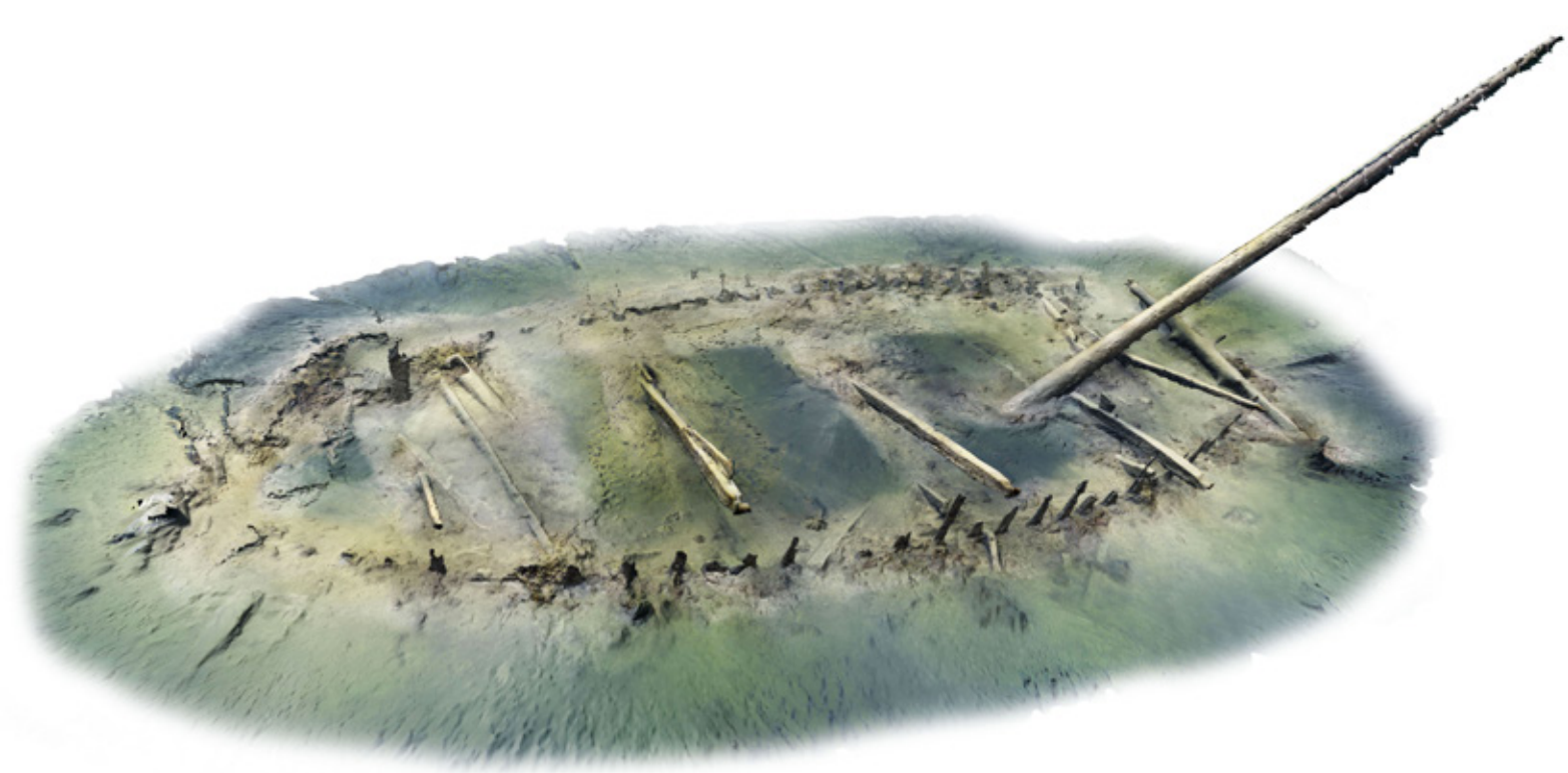
Fotogrammetribild av det medeltida vraket vid Nåttarö. Fartyget ligger med babordssidan djupt nedsjunken och däcksbalkarna pekande snett upp ur botten. Notera den bevarade masten (Statens maritima museer).
