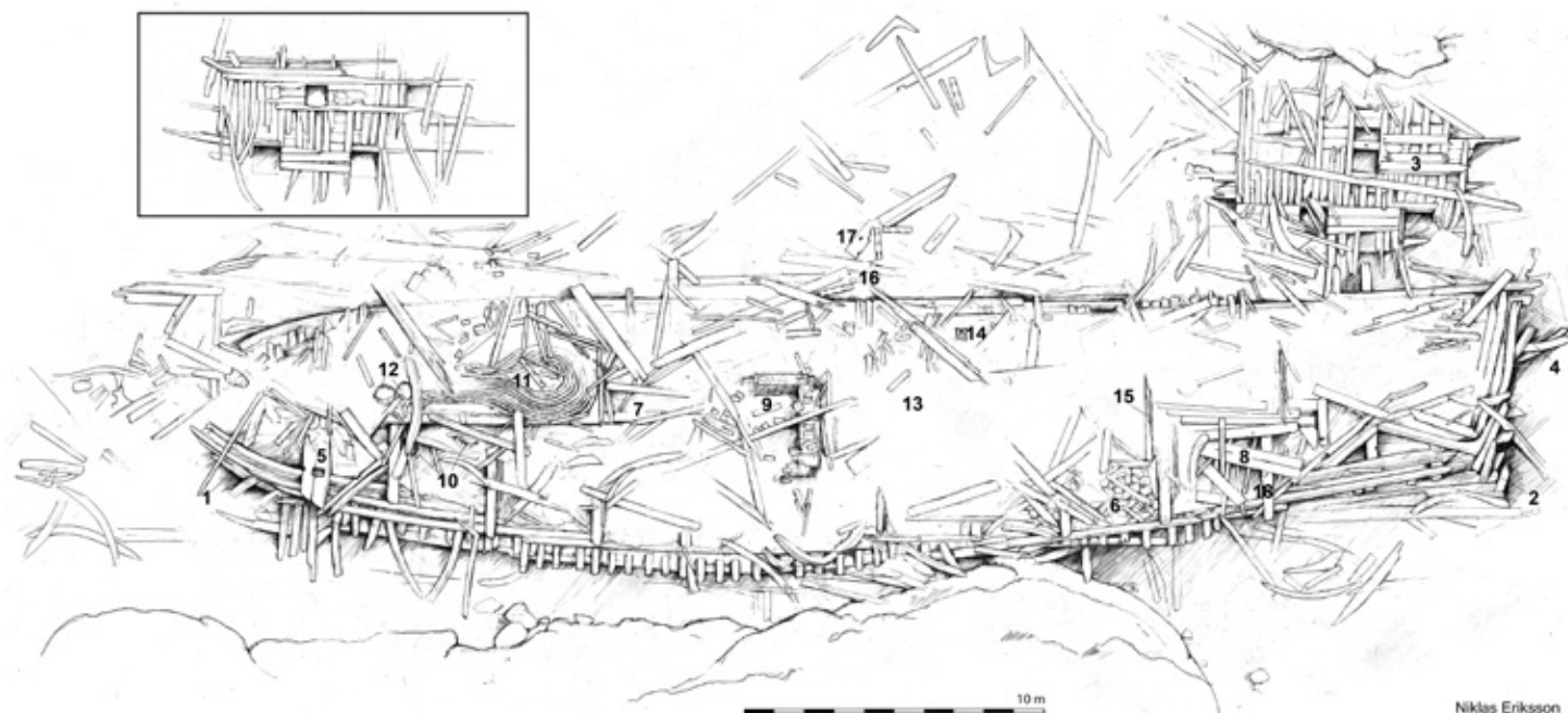
Riksäpplets vrakplats sedd i plan med fören pekande åt vänster. Trots den hårdhända hanteringen finns förvånansvärt mycket kvar av skeppet som vilar på styrbordssidan. Illustration: Niklas Eriksson.
